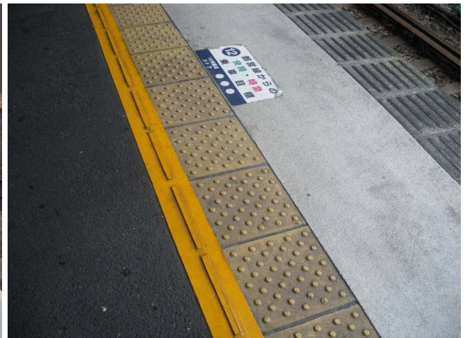
京浜急行 品川駅ホーム(東京寄り) 笠石B～点字B間の表層材:KC-11 内方表示:KC工法 施工 2013年3月
