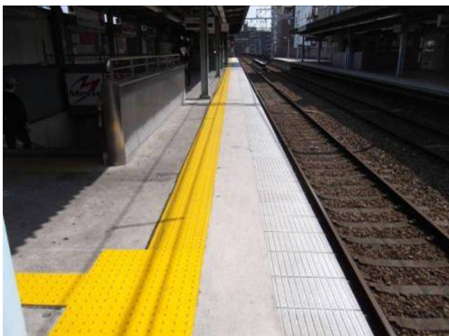
京浜急行 大森海岸駅 内方表示～点字タイル(型枠式カラータイル)および点字タイルと笠石の間 施工 2013年3月
