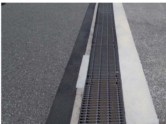
写真3. 側溝際の段差修正 左側下地:密粒アスファルト舗装 右側下地:半たわみ性アスファルト舗装
